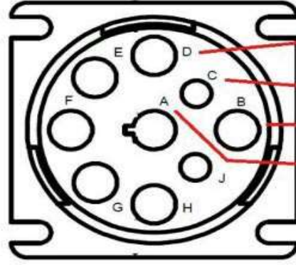
Ford Cargo 1846 - 460 PS - 9 pinli Arıza tespit soketi
